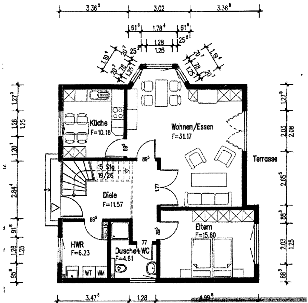
Grundriss EG 30
