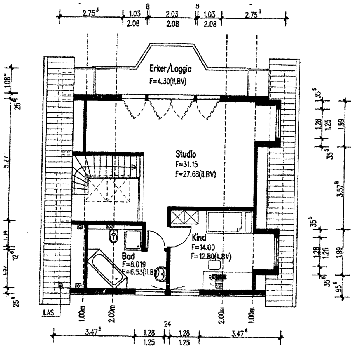
Grundriss OG 30
