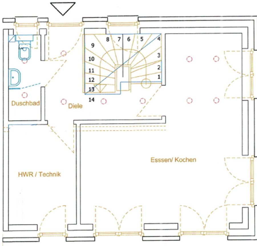
ERDGESCHOSS
