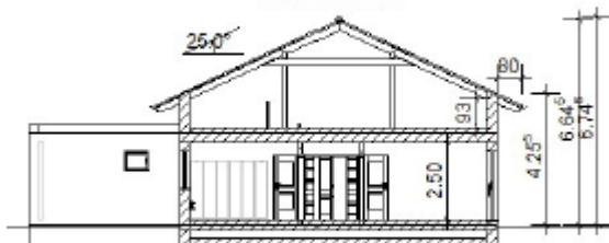
Schnitt A--A
