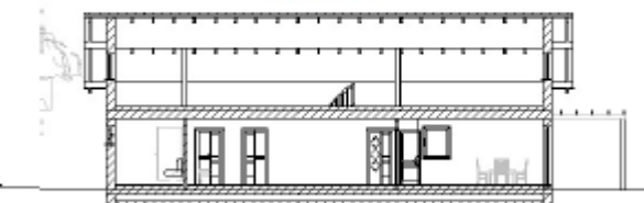
Schnitt B--B
