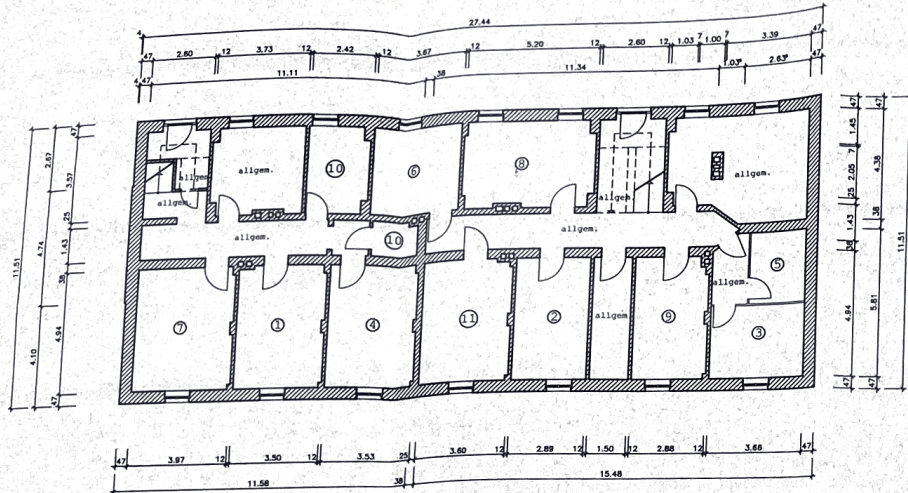
Kellergrundriß
