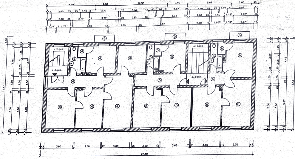
1. Obergeschossgrundriß
