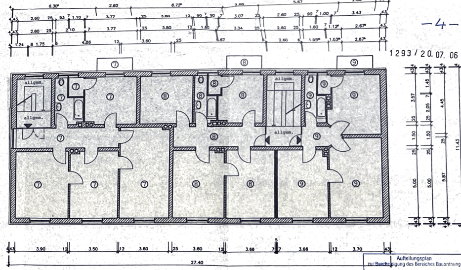
2. Obergeschossgrundriß
