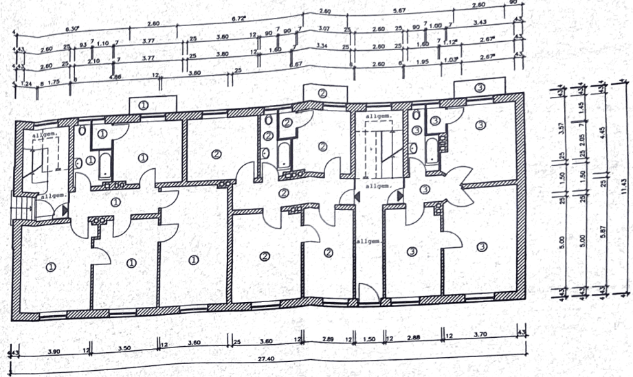
Erdgeschossgrundriß
