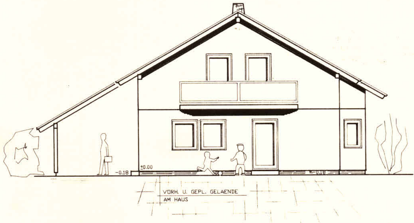
NORD—WEST ANSICHT
