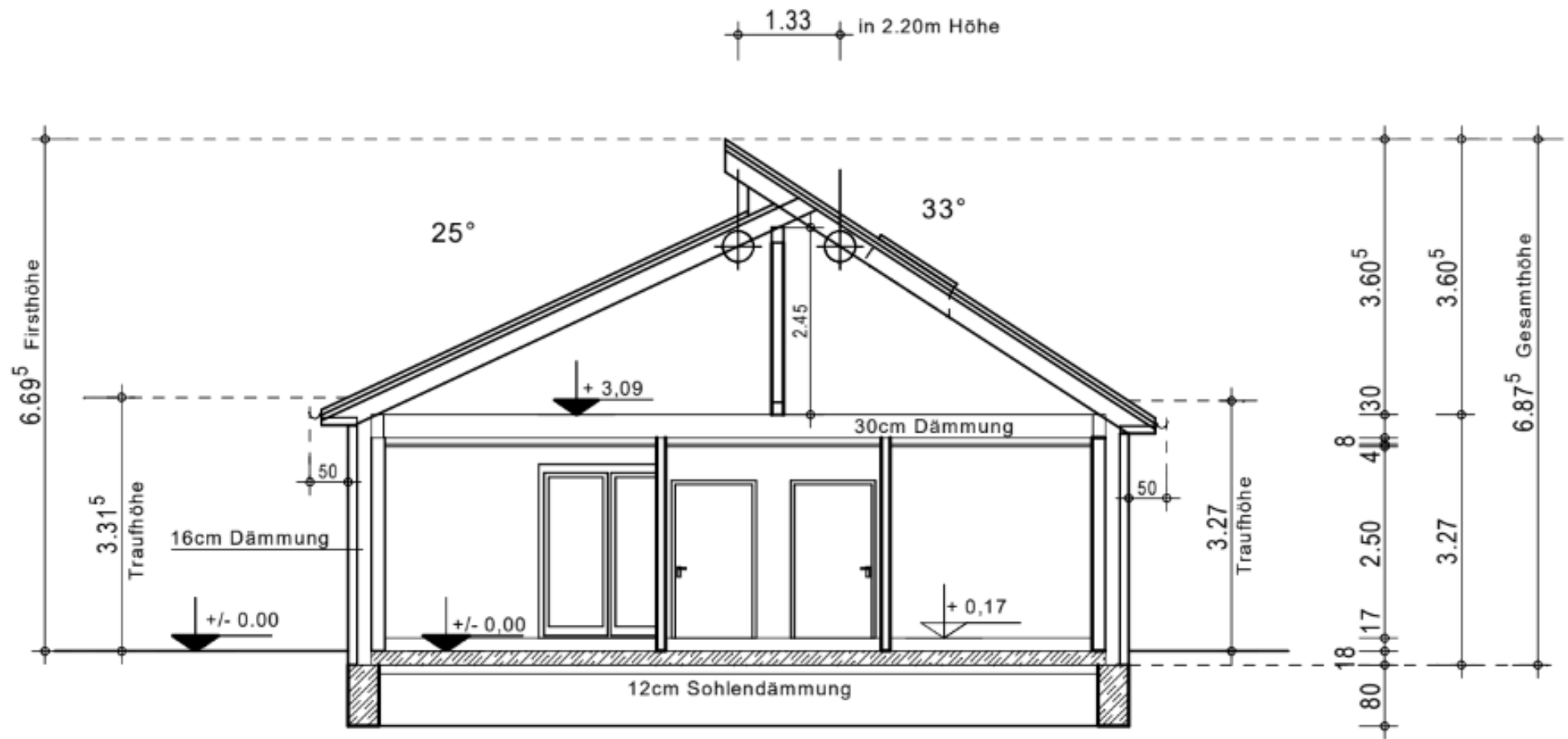
Schnitt A-A
