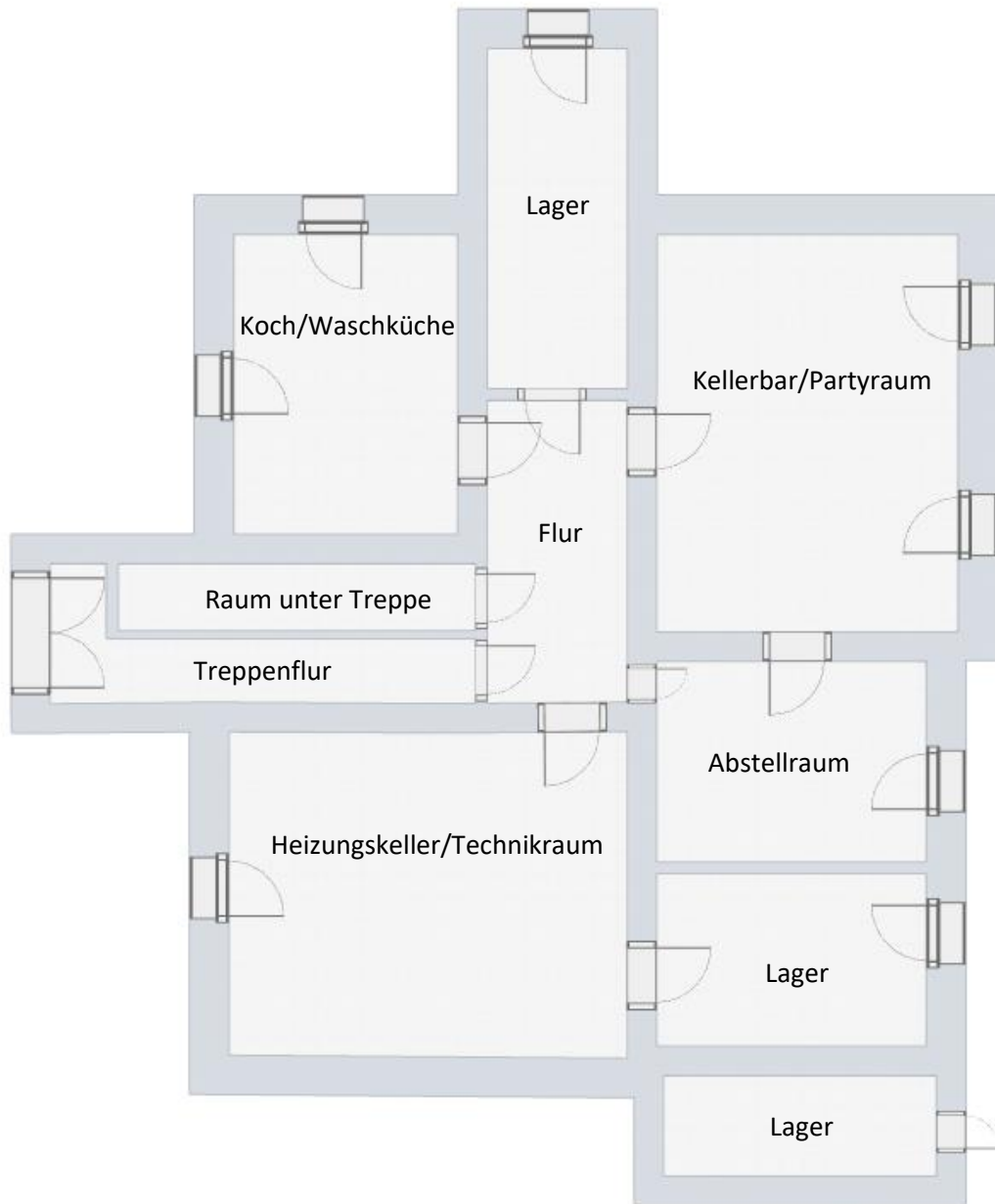
Fachwerkhaus Kellergeschoss
