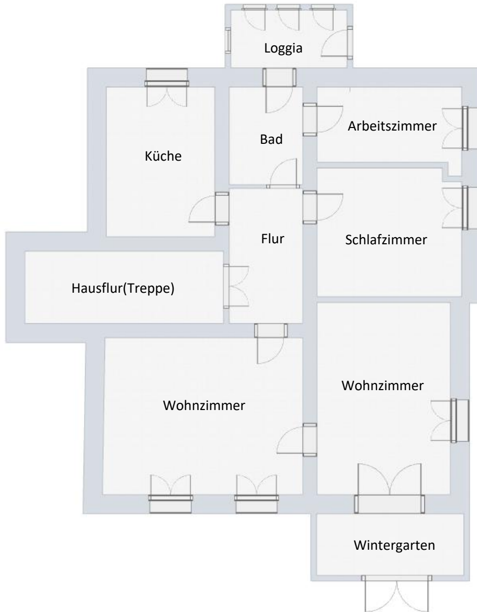
Fachwerkhaus Erdgeschoss
