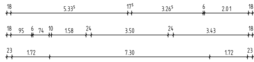
1.OBERGESCHOSS
