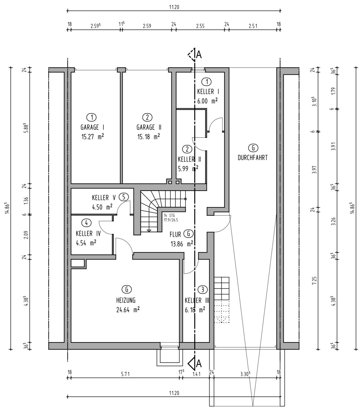
KELLERGESCHOSS
