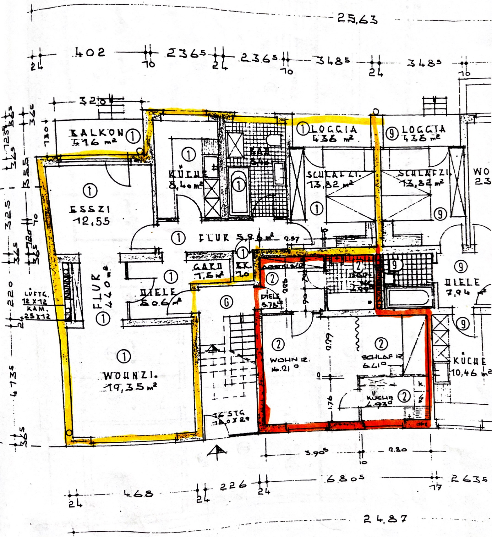
ERDGESCHOSS M-1:100
