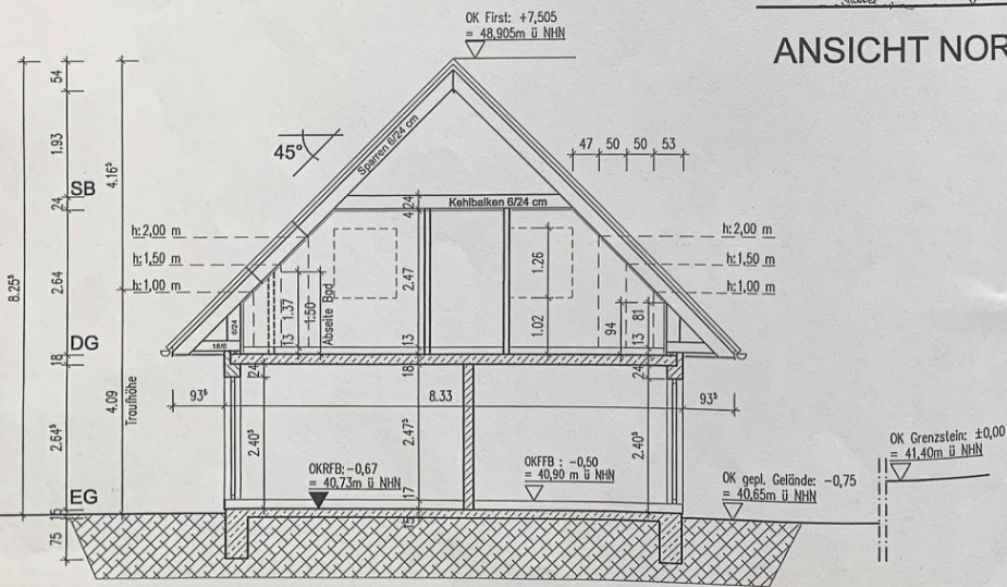
SCHNITT
