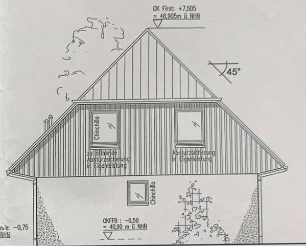
ANSICHT NORDOSTEN
