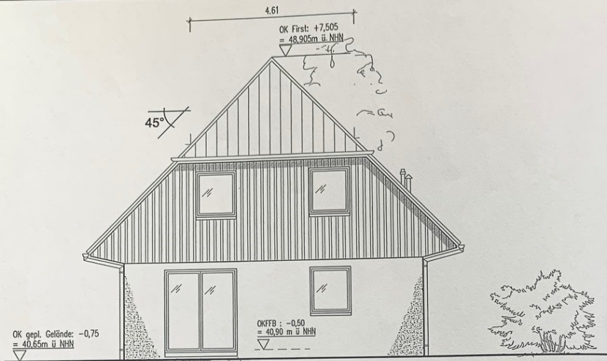
ANSICHT SÜDWESTEN
