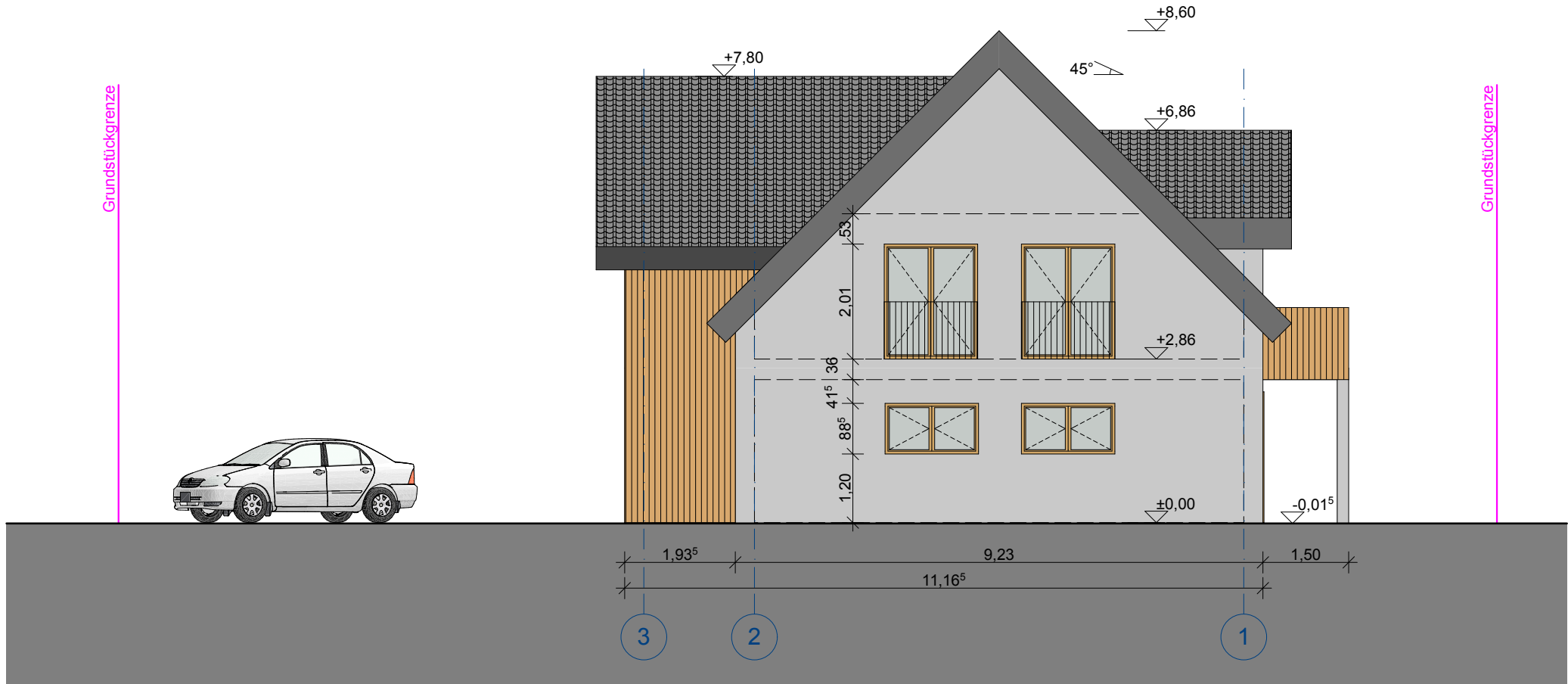
ANSICHT VON WESTEN_M 1:100
