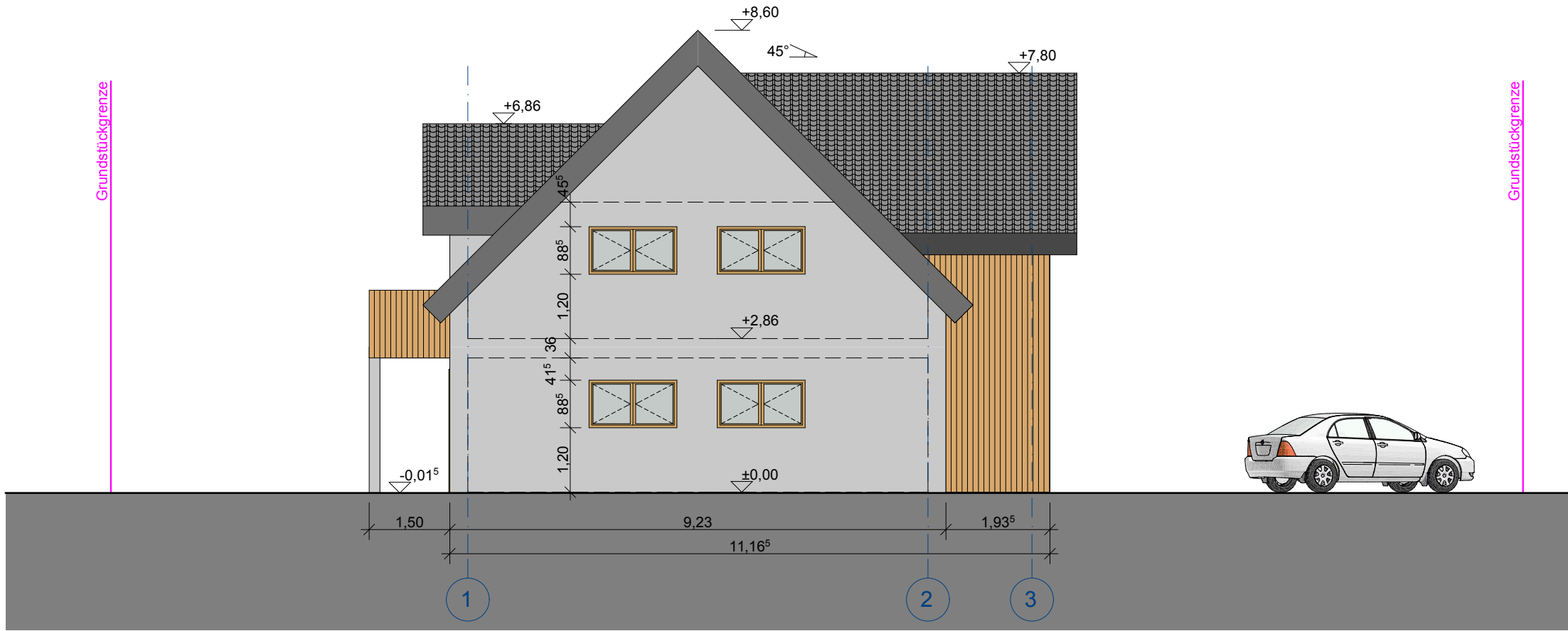
ANSICHT VON OSTEN_M 1:100
