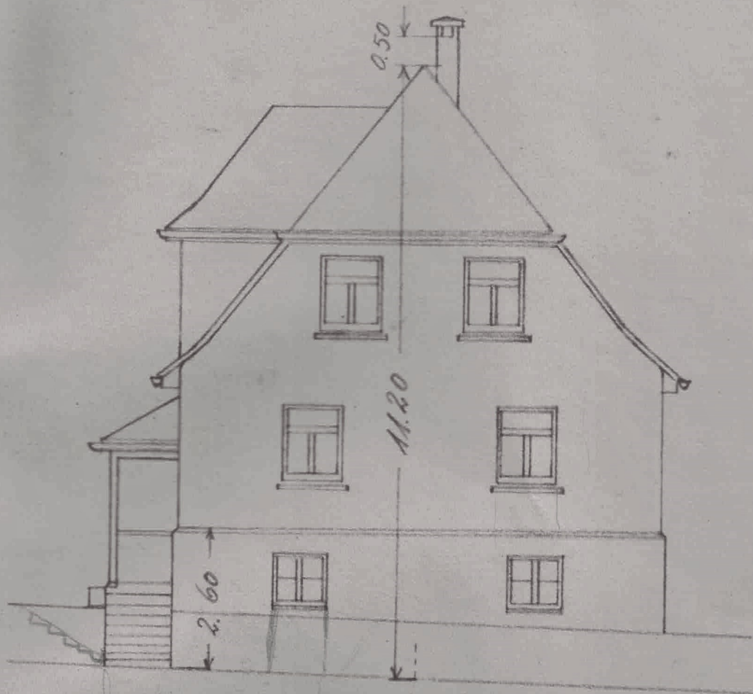
Ansicht - Straßenseite.
