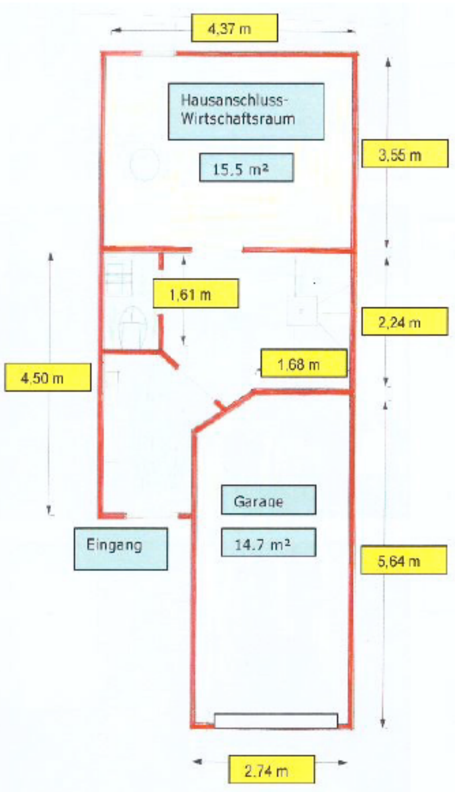
Grundriss UG
