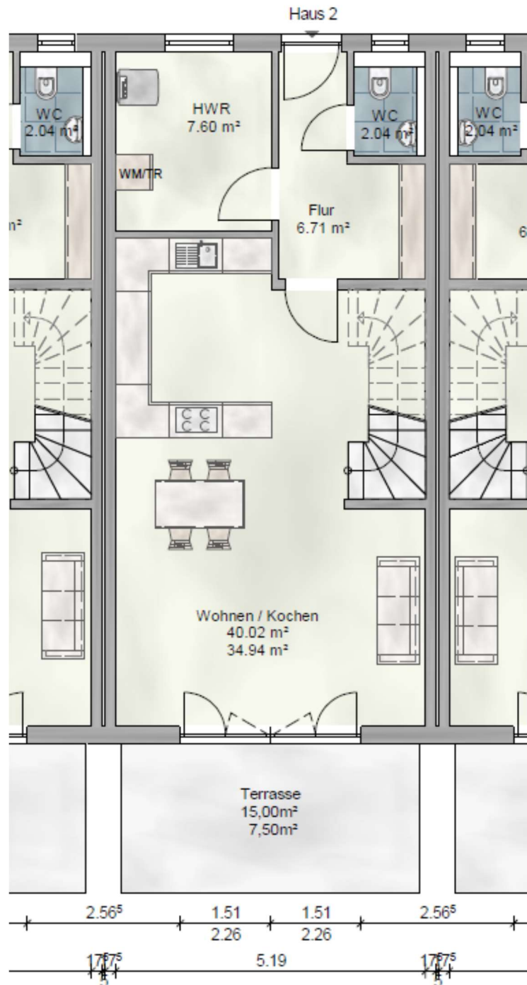
Grundriss EFH Mittelhaus Erdgeschoss - variabel
