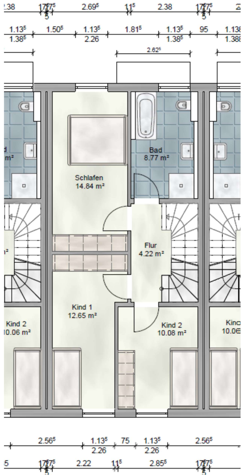
EFH Mittelhaus Grundriss OG - variabel
