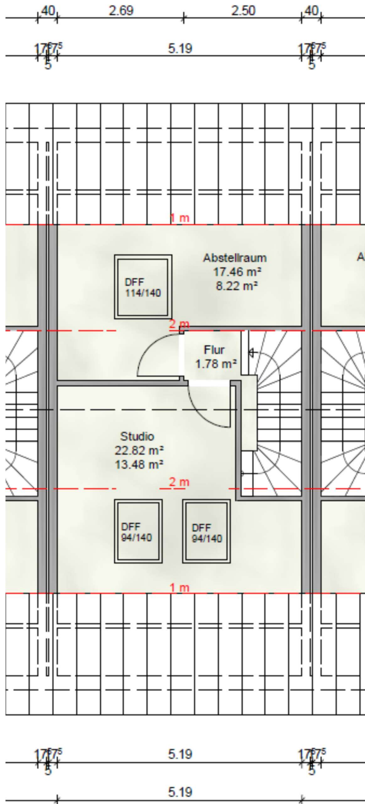
EFH Mittelhaus Grundriss DG - variabel
