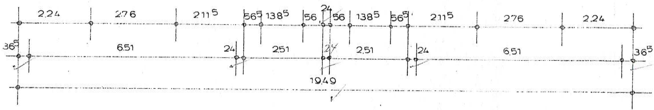
ERDGESCHOSS BZW. OBERGESCHOSS
