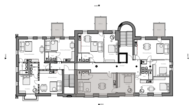
Übersichtsplan Ebene E3
