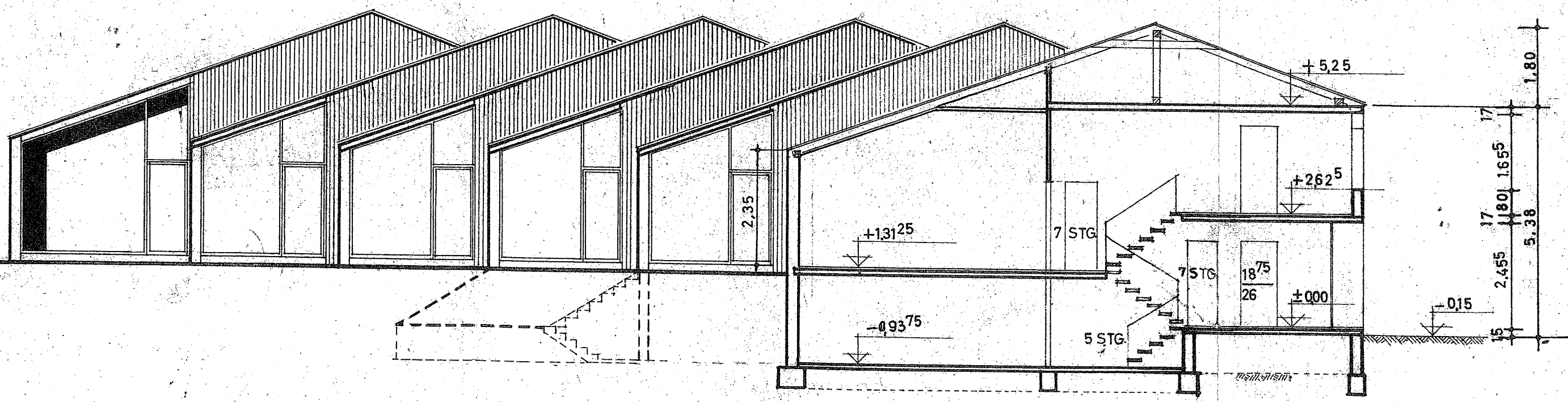
SCHNITT A-A
