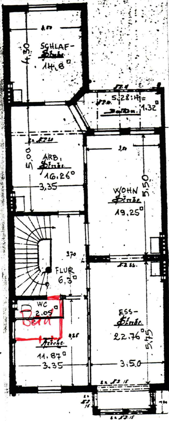
I. Obergeschoss
