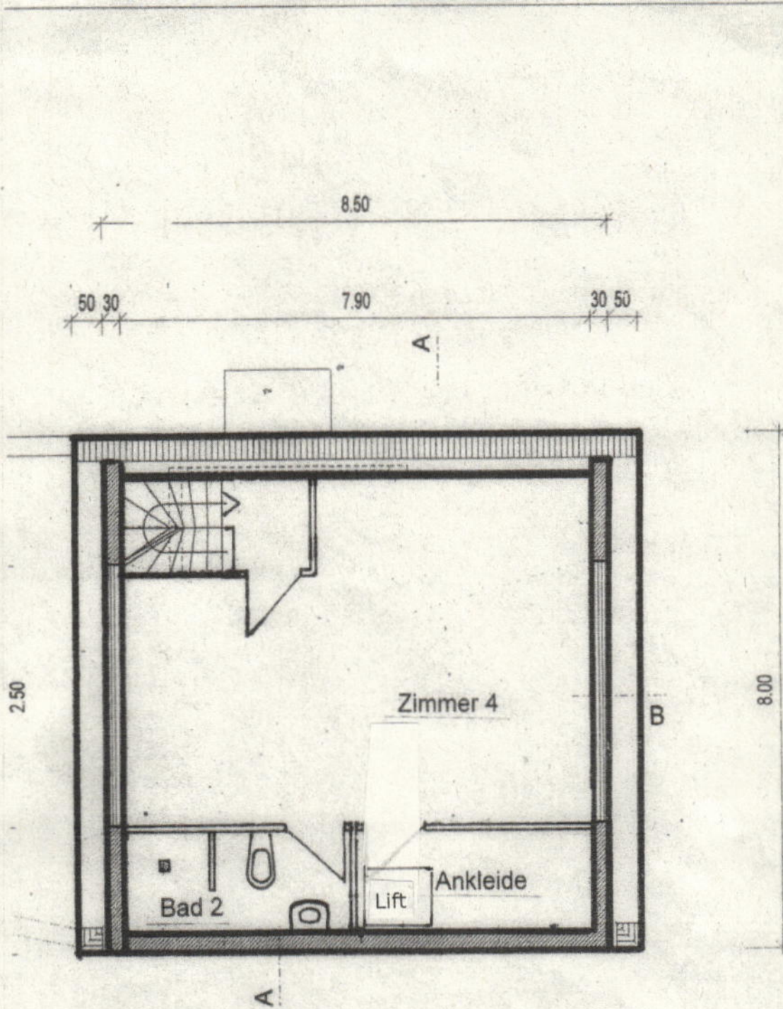
2. OBERGESCHOSS
