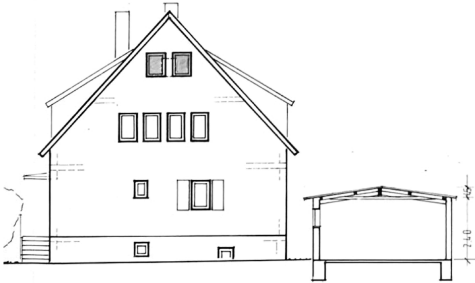
Ansicht Nord
