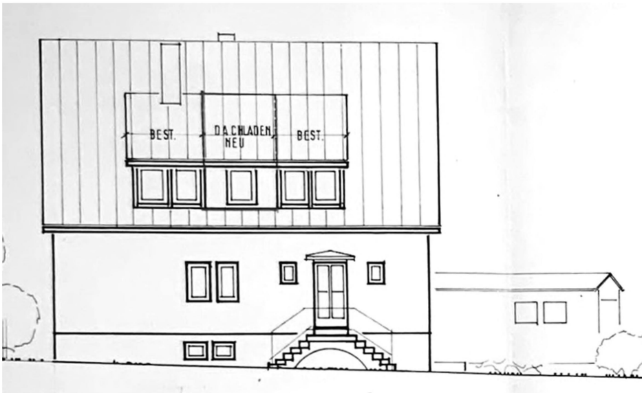
Ansicht Ost
