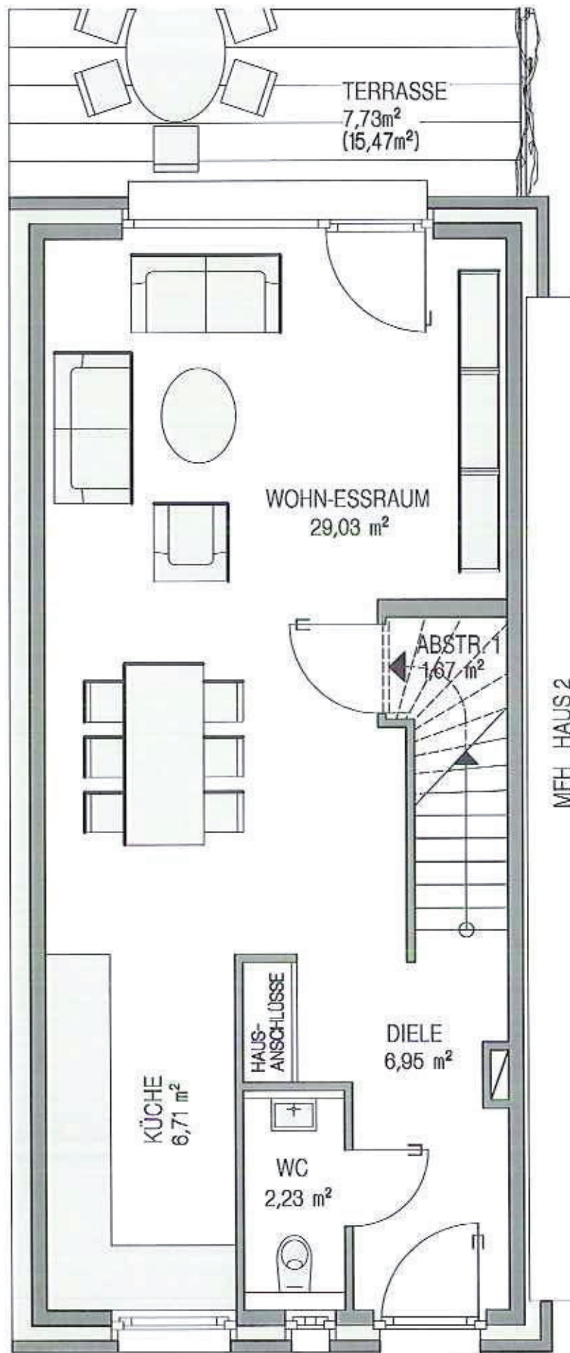
ERDGESCHOSS M.1:50 HAUS 1 (HAUS 6 SPIEGELBILDLICH) BV: LÜRRIP, GERTHMÜHLENWEG
