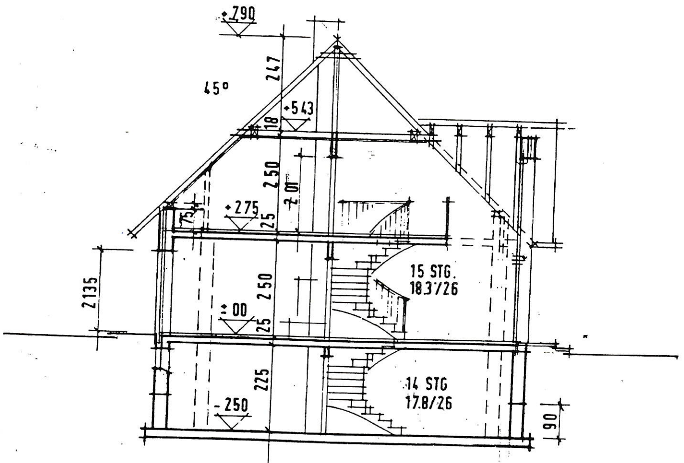
SCHNITT A-A
