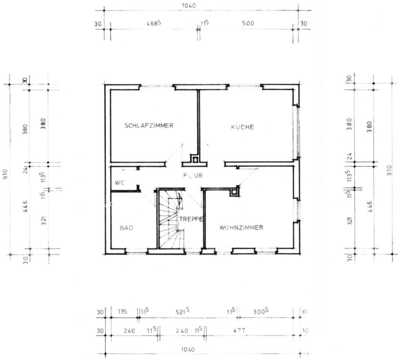
Grundriss Obergeschoss
