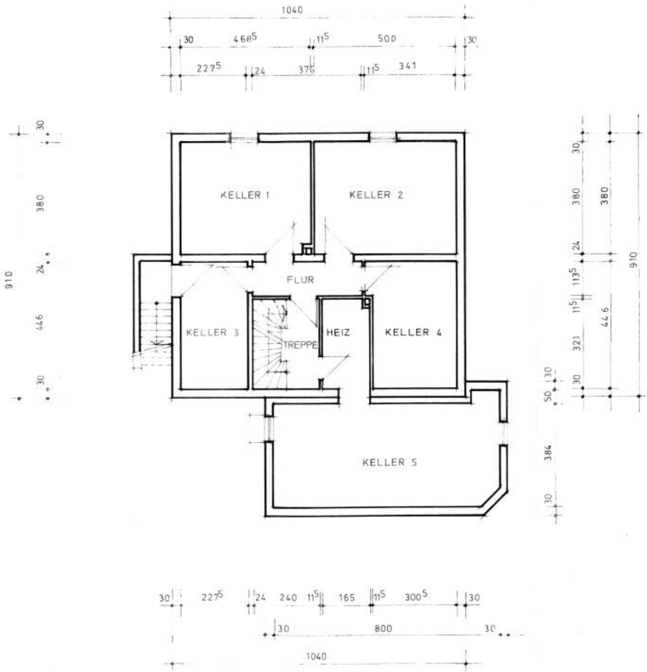
Grundriss Kellergeschoss
