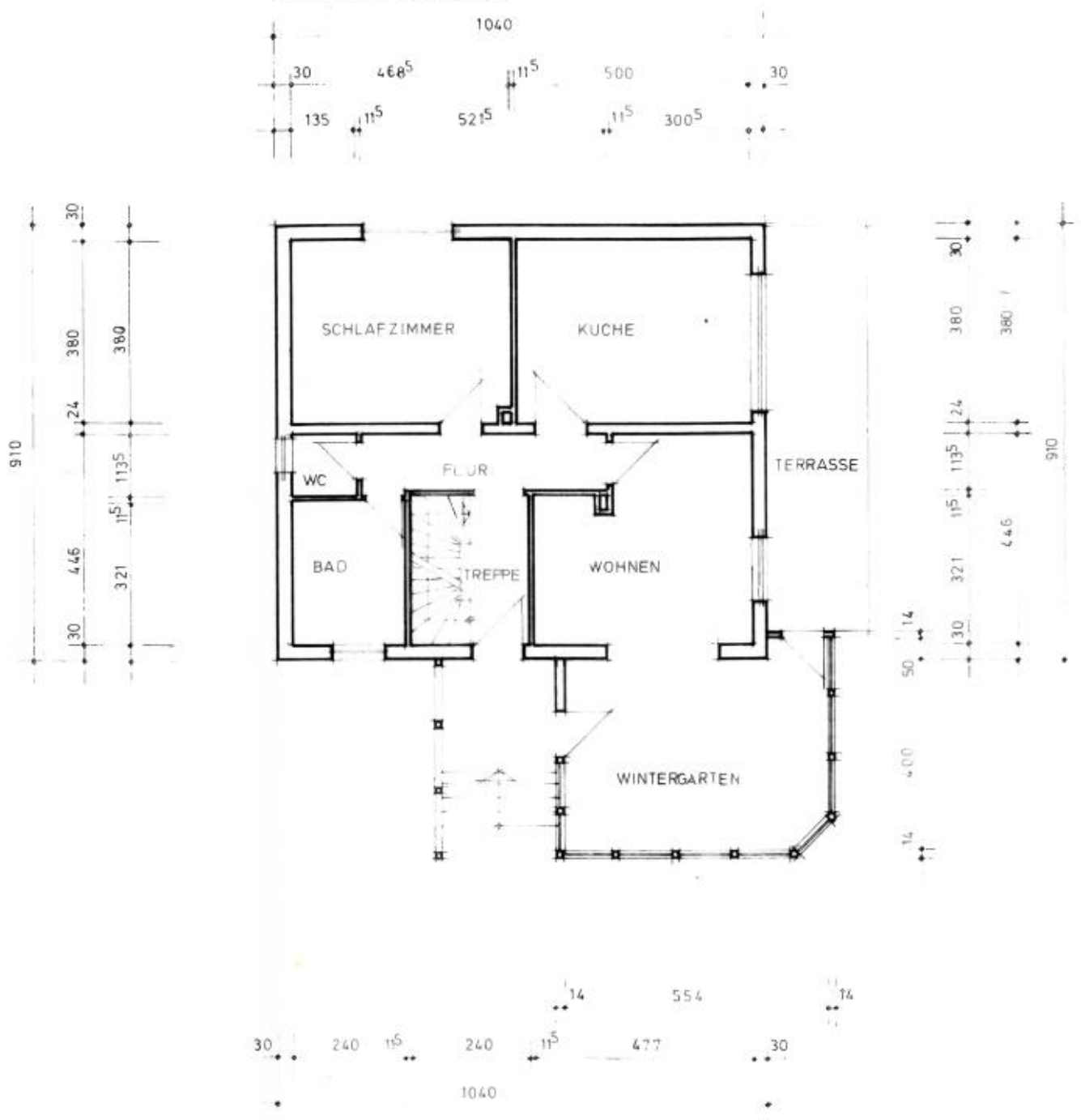
Grundriss Erdgeschoss
