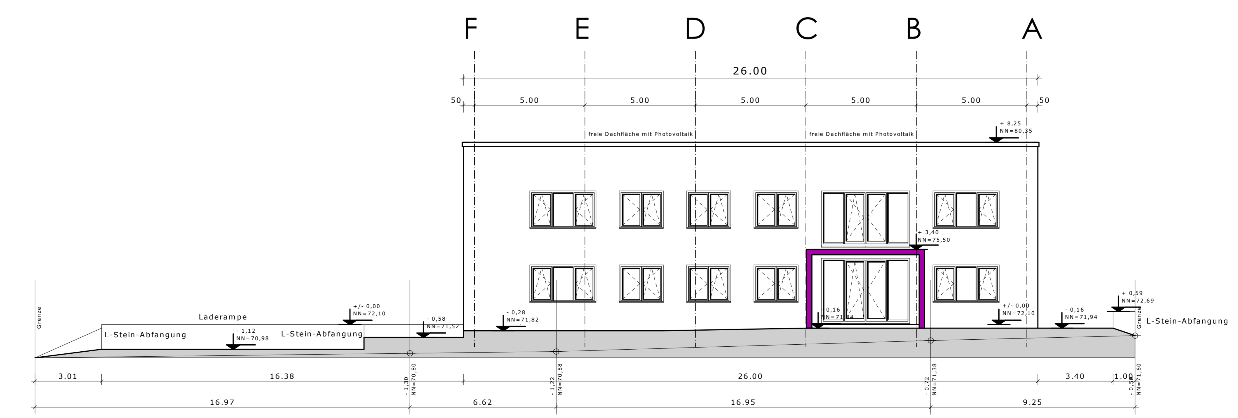
ANSICHT SÜD
