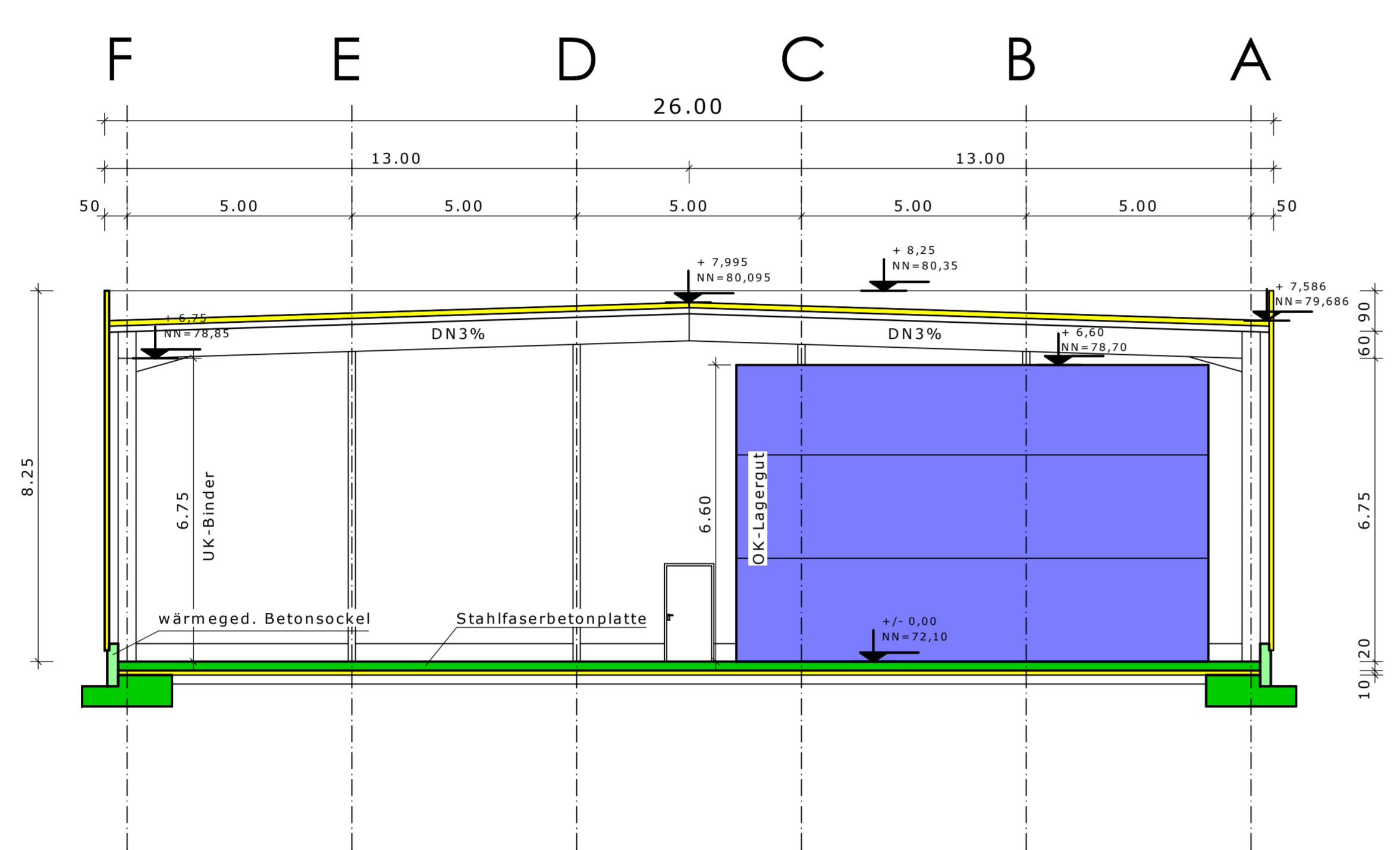
SCHNITT A-A
