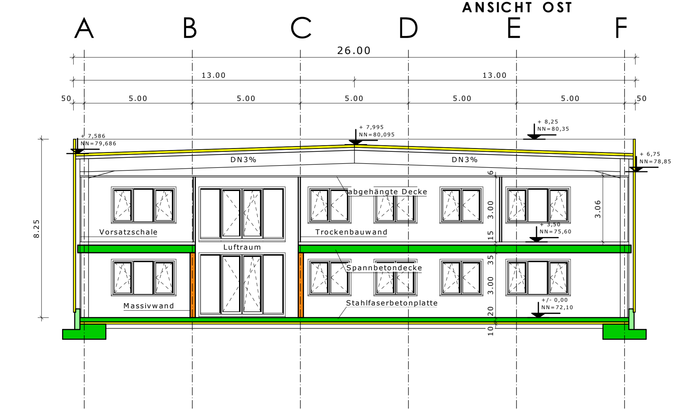
SCHNITT B-B
