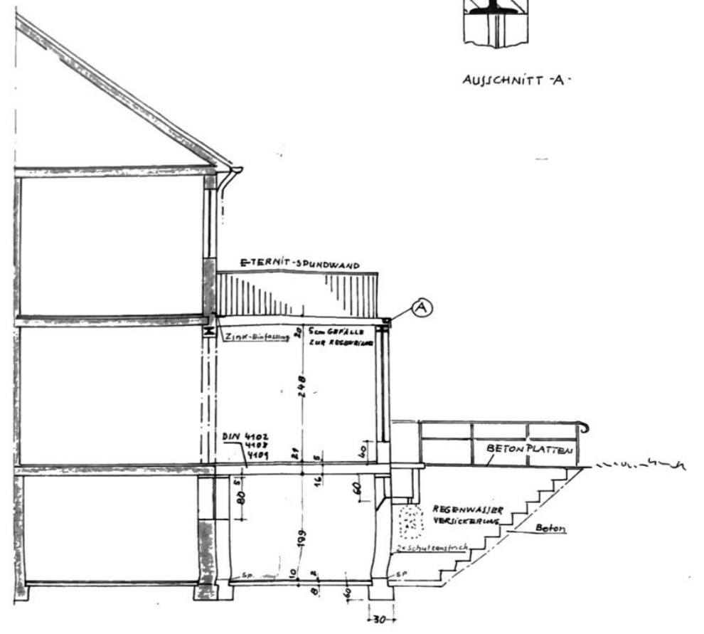
SCHNITT I
