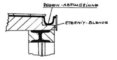
AUSSCHNITT -A-
