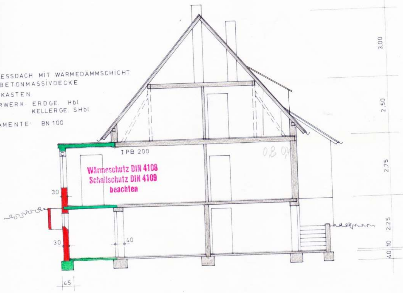
SCHNITT A-B
