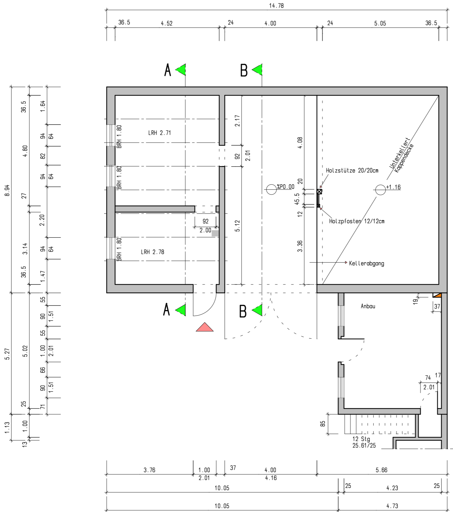
Grundriss EG
