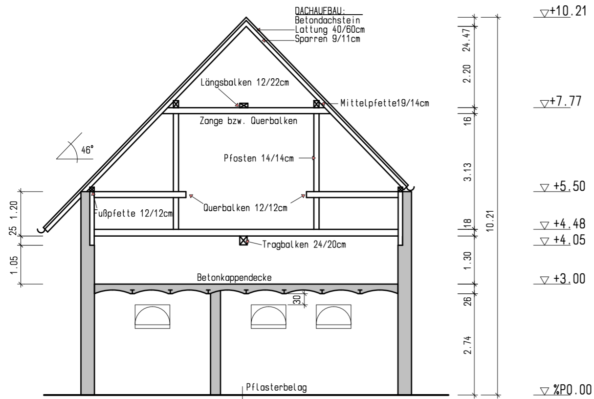
Schnitt A-A Bestand
