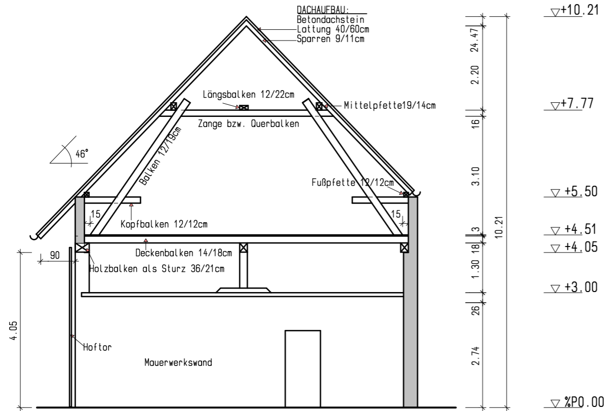
Schnitt B-B Bestand
