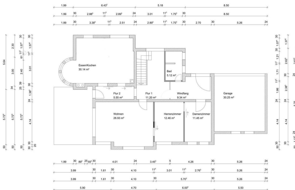
Grundriss EG, bemaßt
