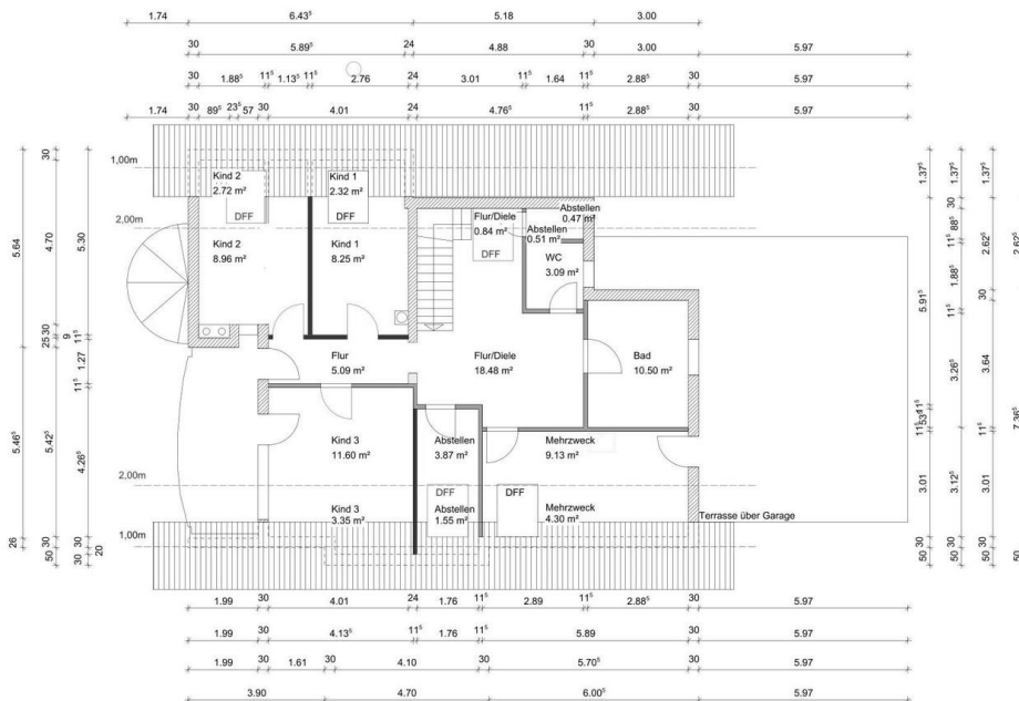
Grundriss OG, bemaßt
