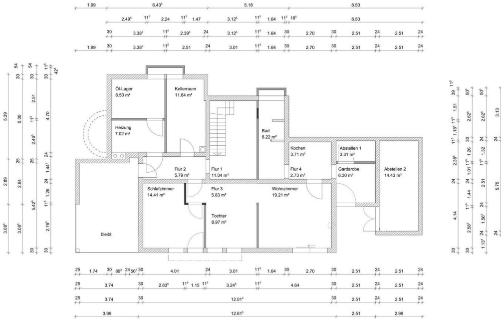
Grundriss UG, bemaßt
