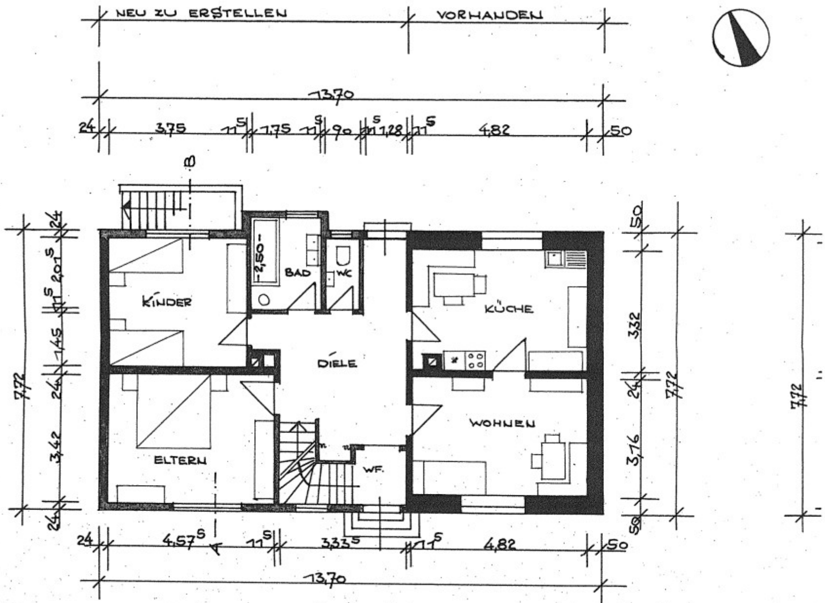
ERDGESCHOSSGRUNDRISS
