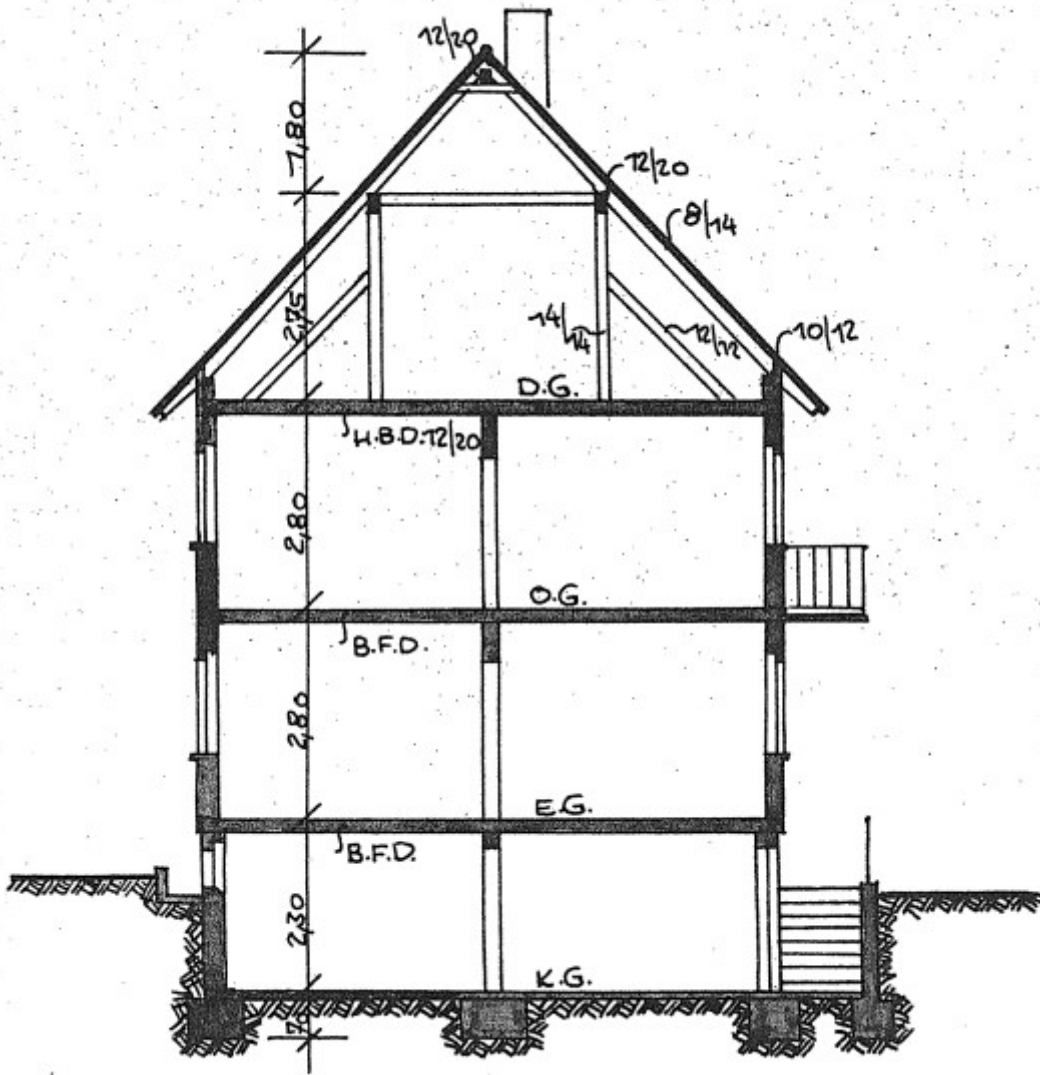
QUERSCHNITT A-B
