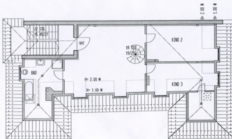
DACHGESCHOSS
