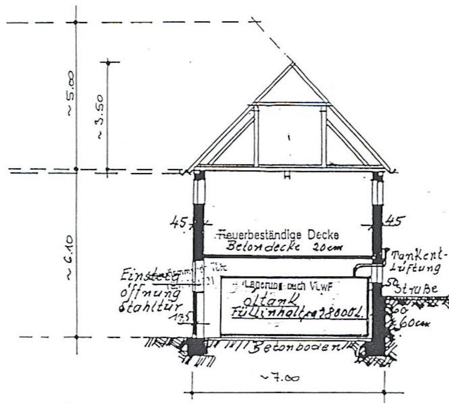
SCHNITT SKIZZE OHNE MASSTAB
