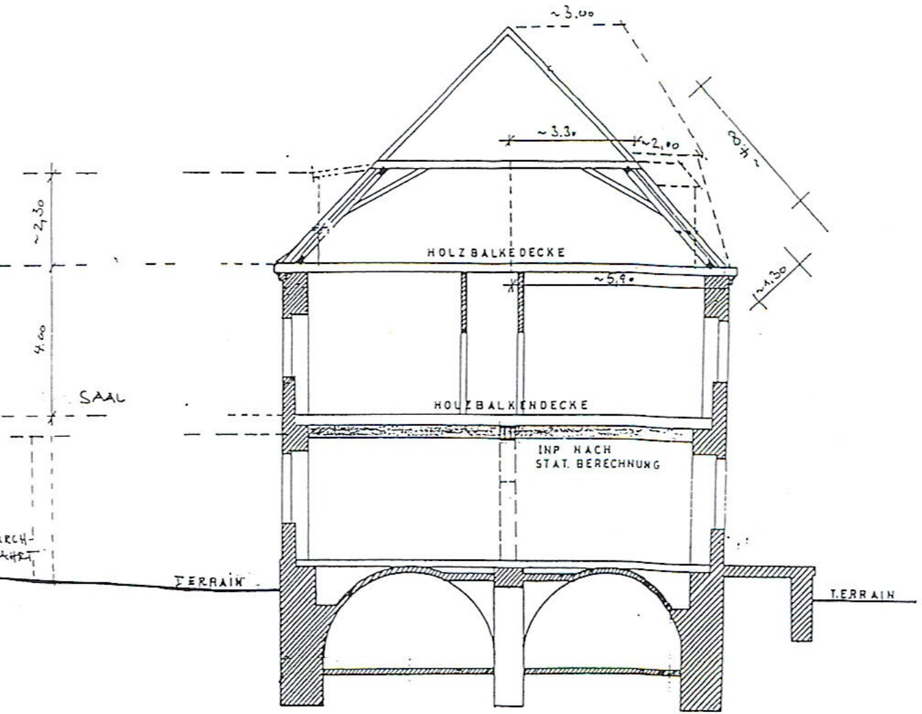
SCHNITT SKIZZE OHNE MASSTAB
