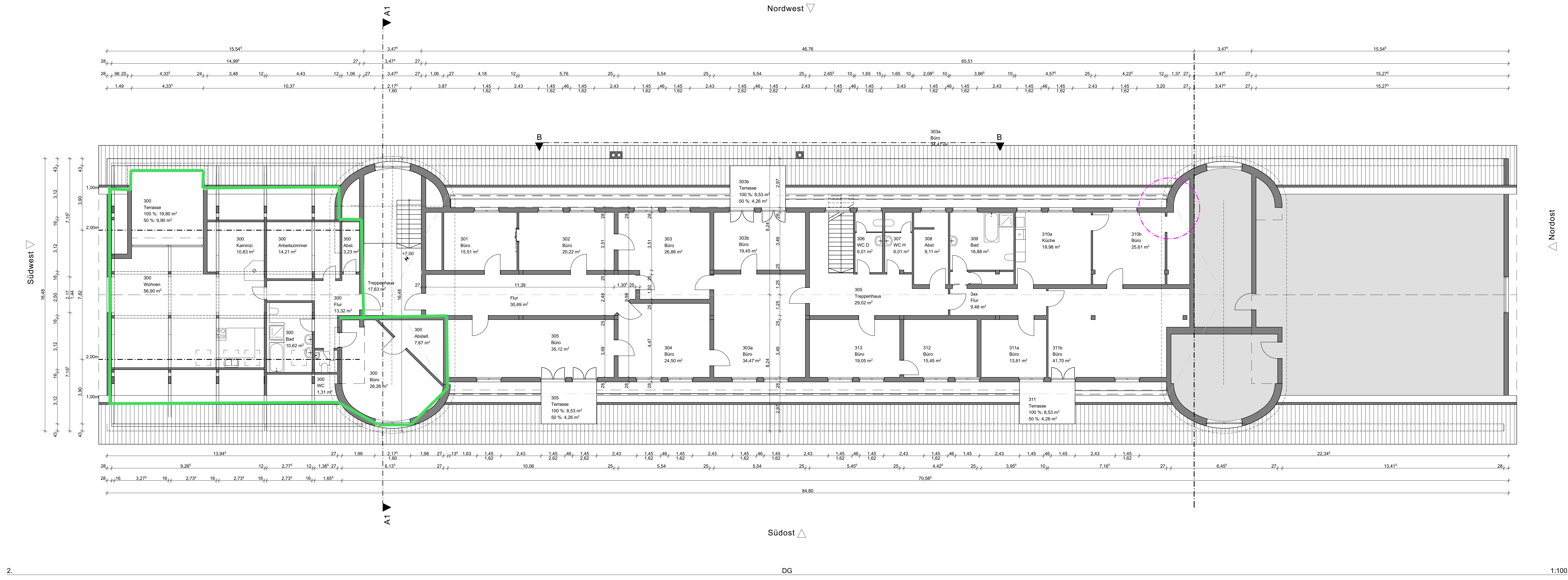
2. DG 1:100
