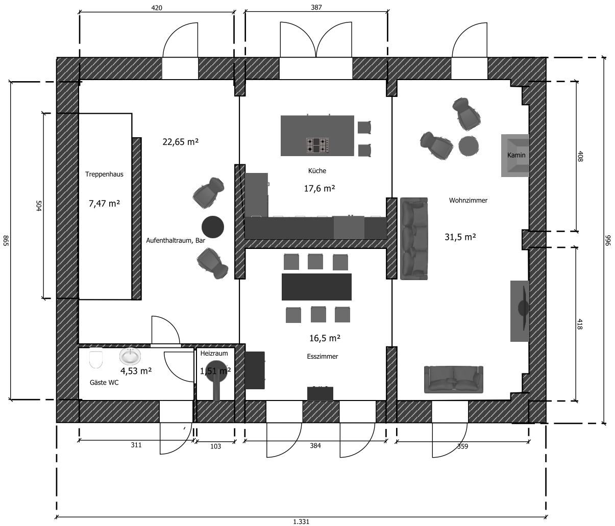
Grundriss 1.Obergeschoss
