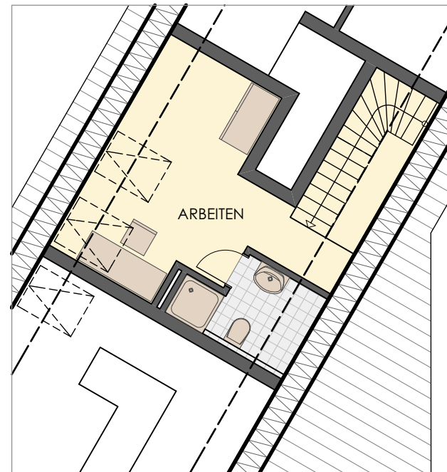
Grundriss SPITZBODEN
