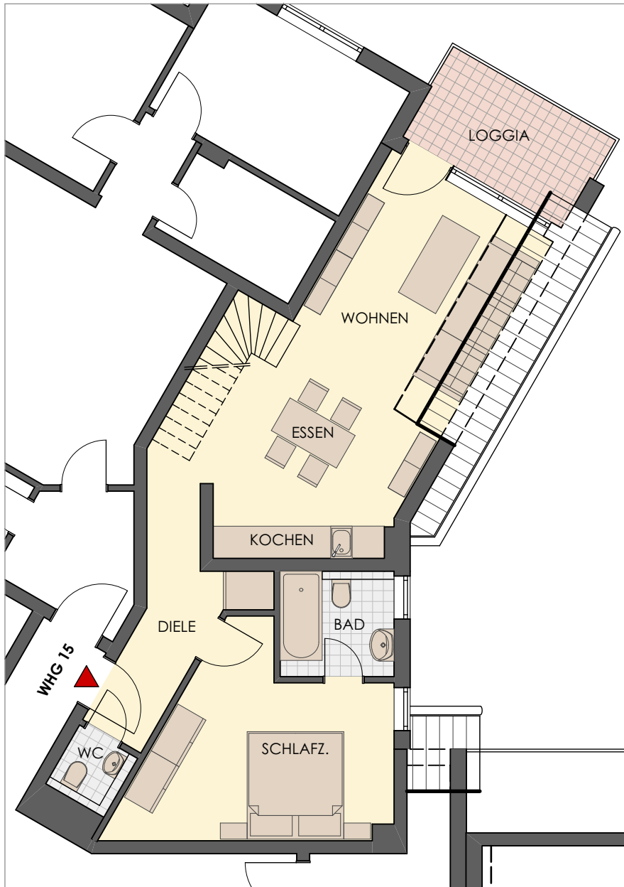
Grundriss DACHGESCHOSS
