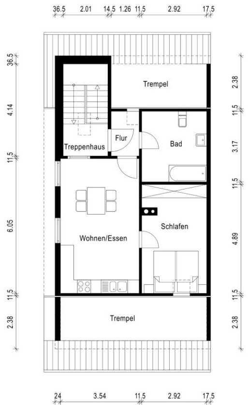
Dachgeschoss
