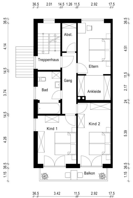
1.Obergeschoss
