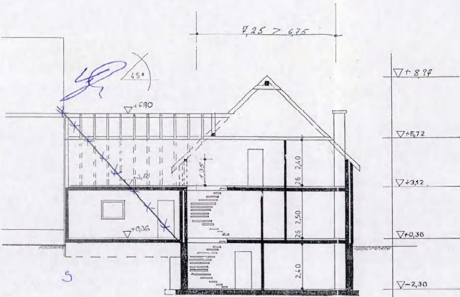
SCHNITT A-A
