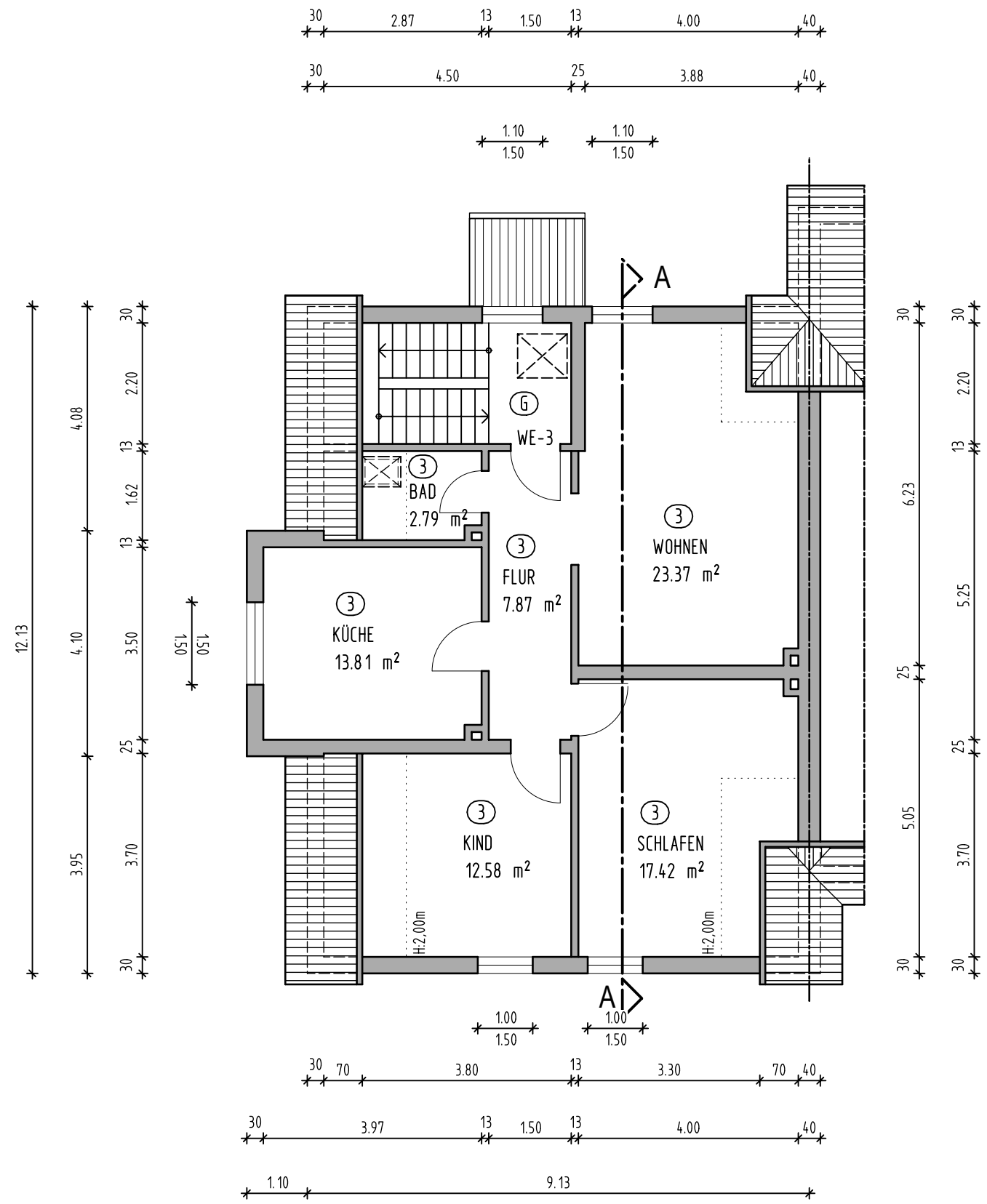
DACHGESCHOSS
