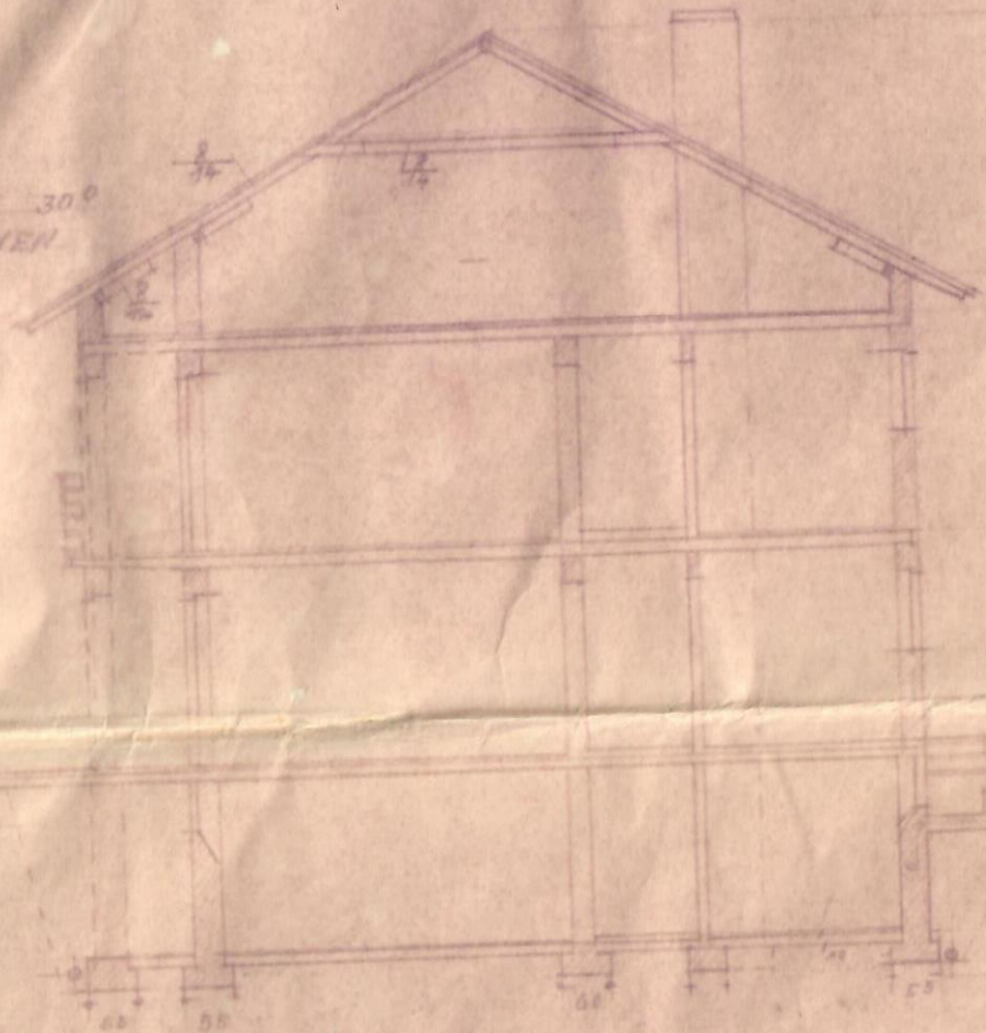
-0 SCHNITT 0-
