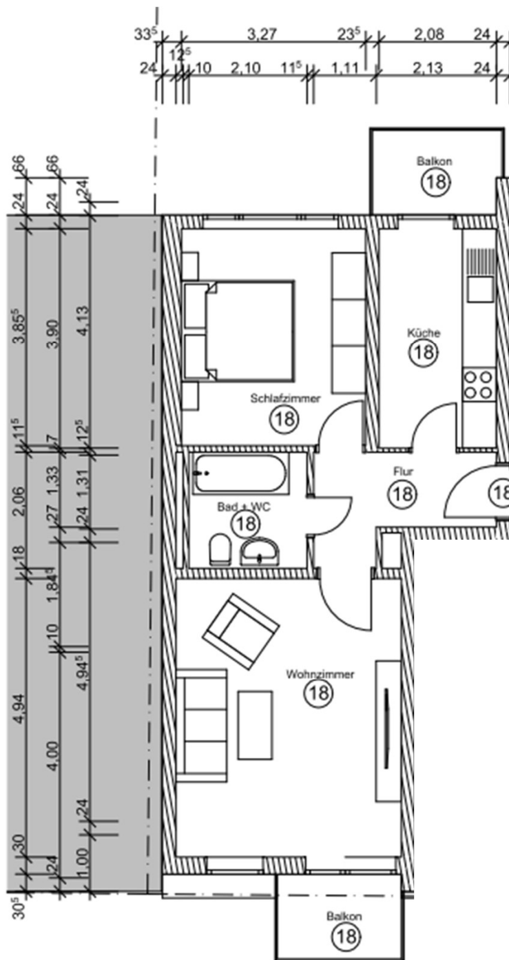
1. OBERGESCHOSS
