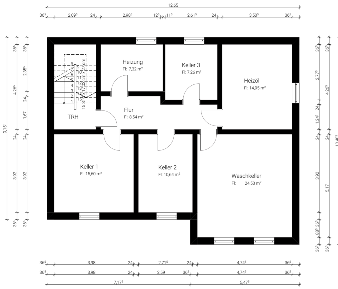
Grundriss KG
