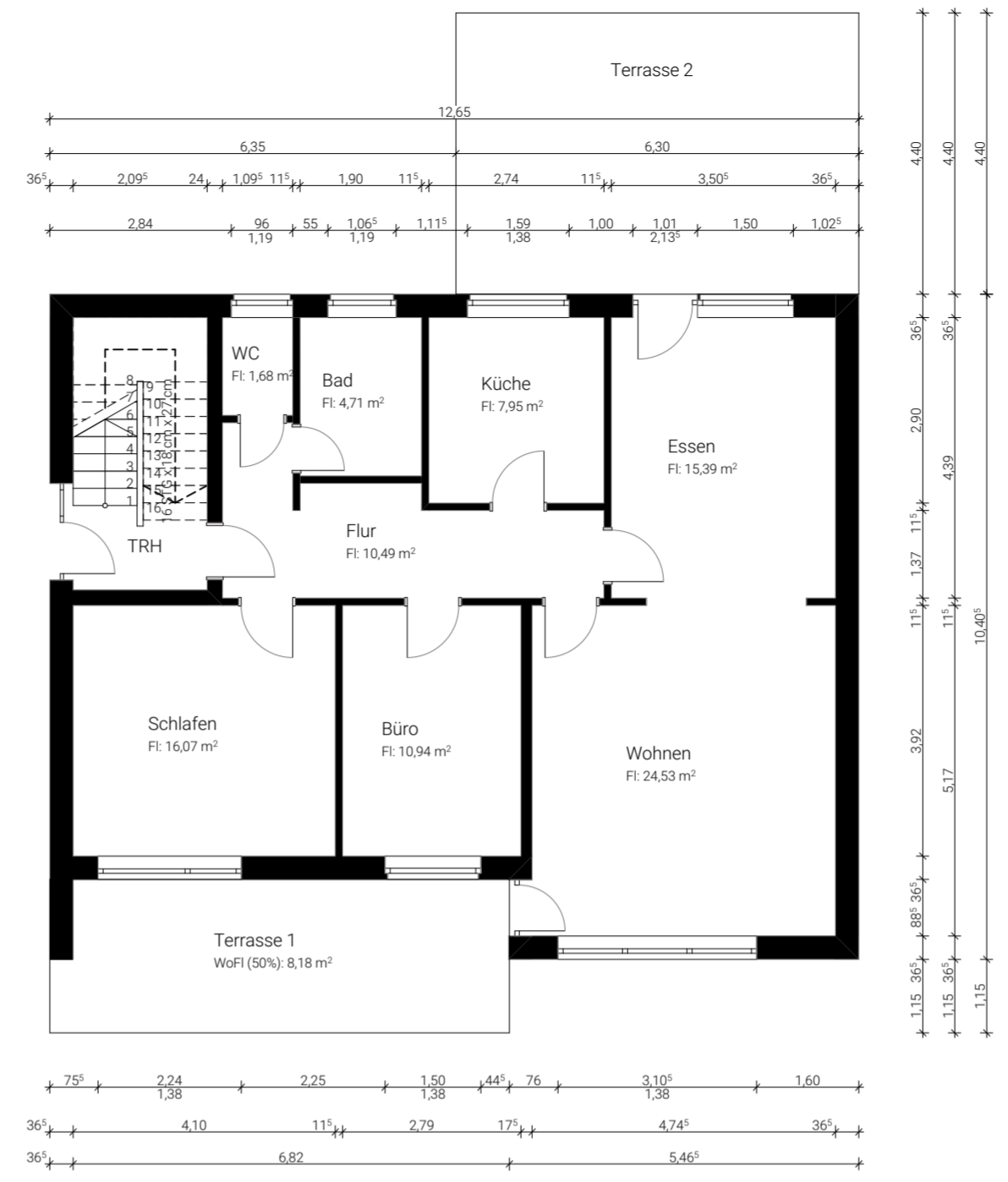
Grundriss EG
