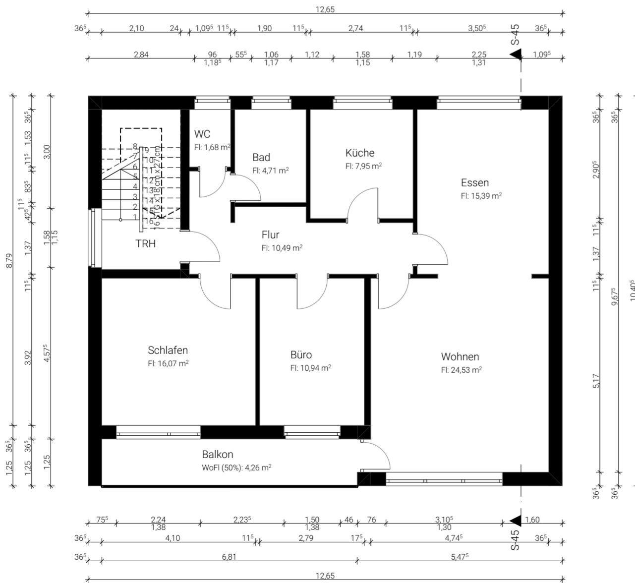
Grundriss 1. OG
