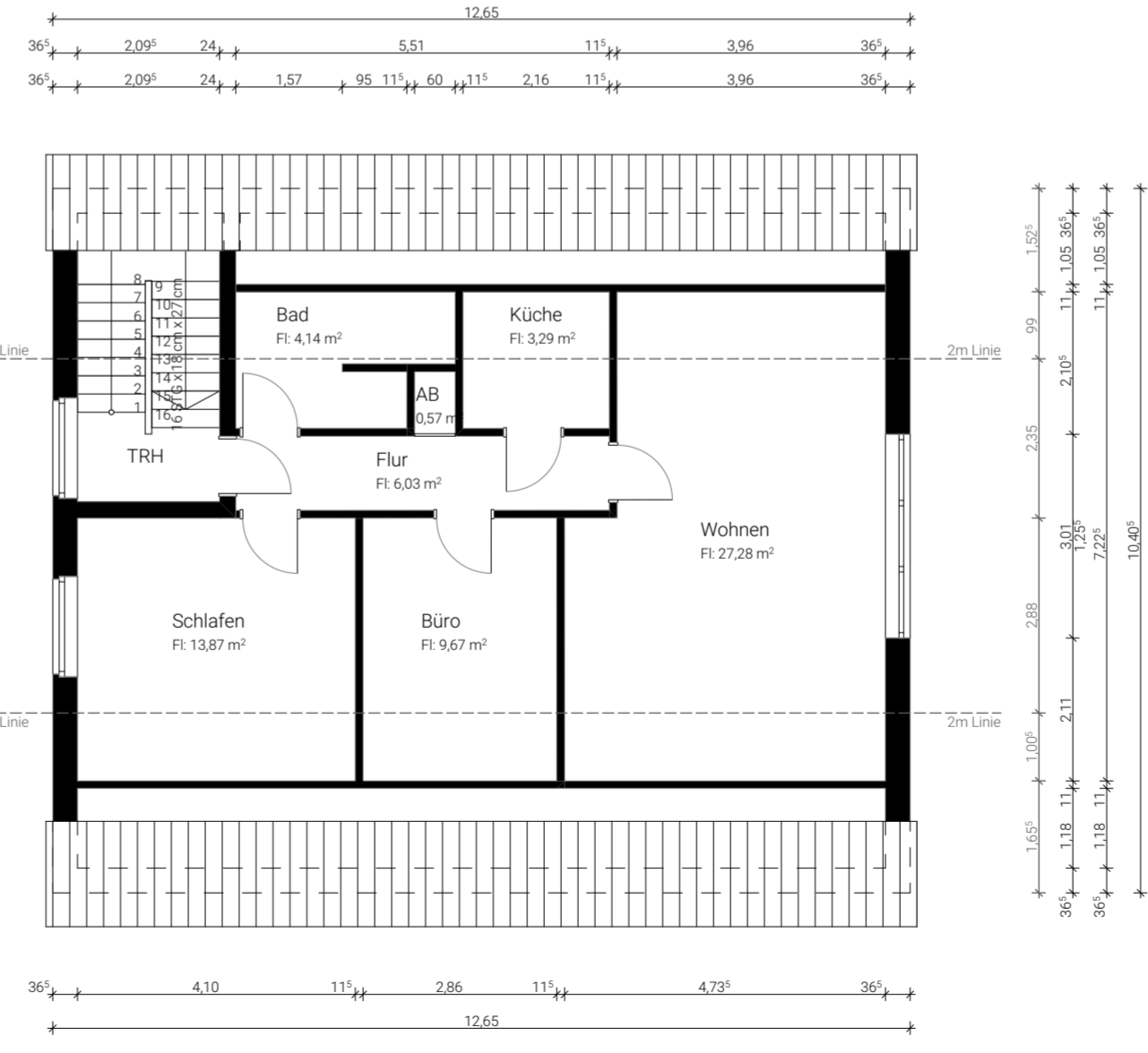
Grundriss DG
