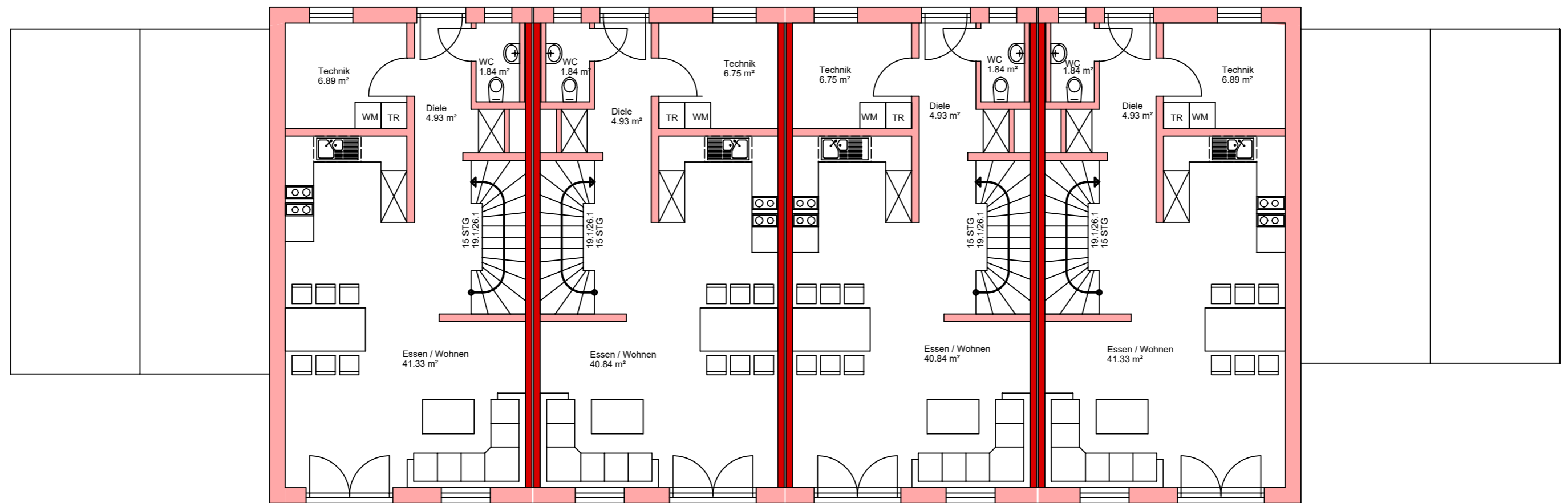
Erdgeschoss
