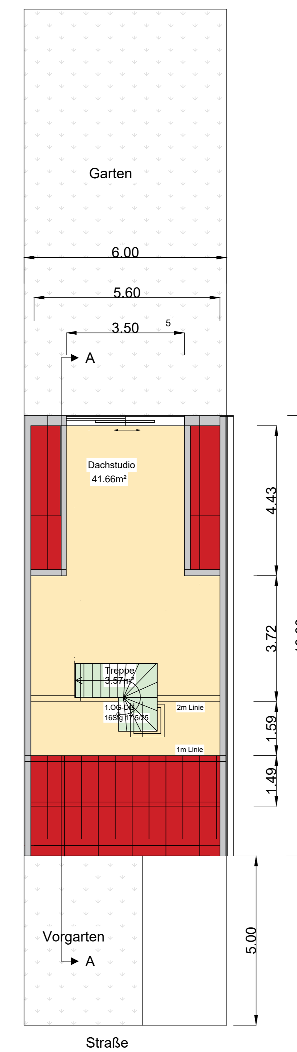
DG 41.66m 2
