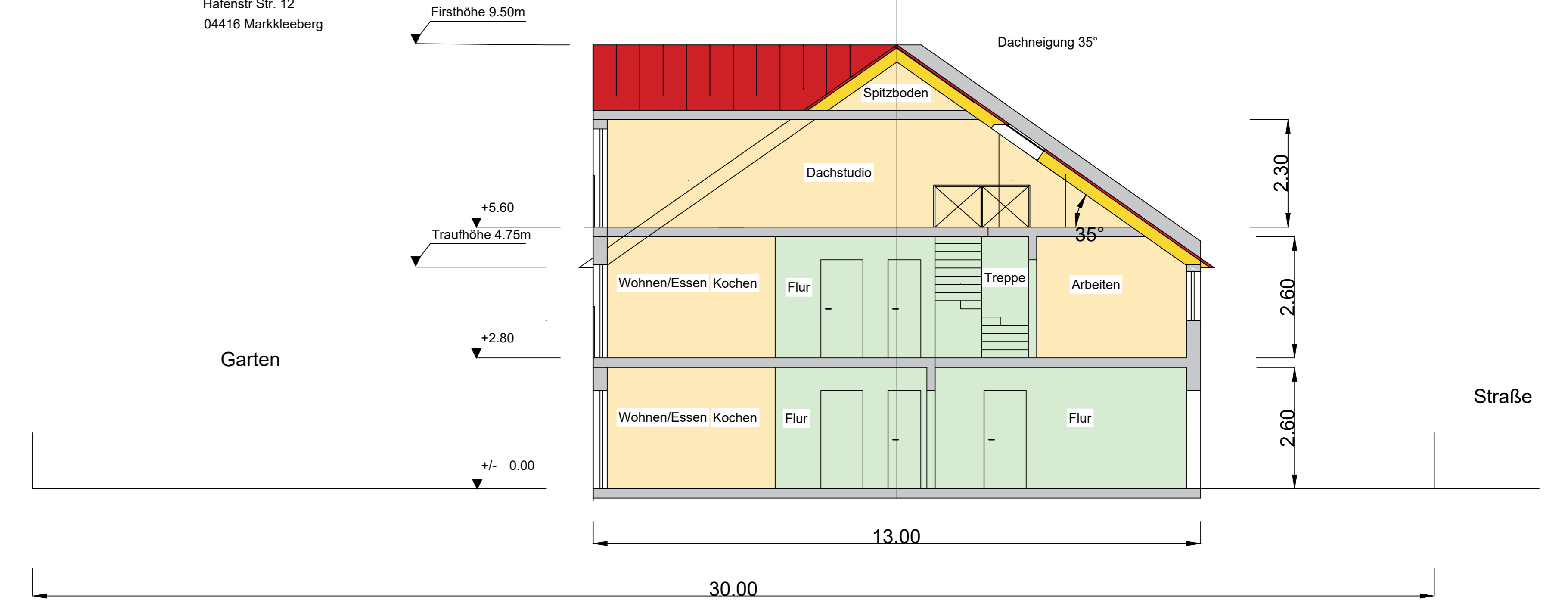
Schnitt A - A
